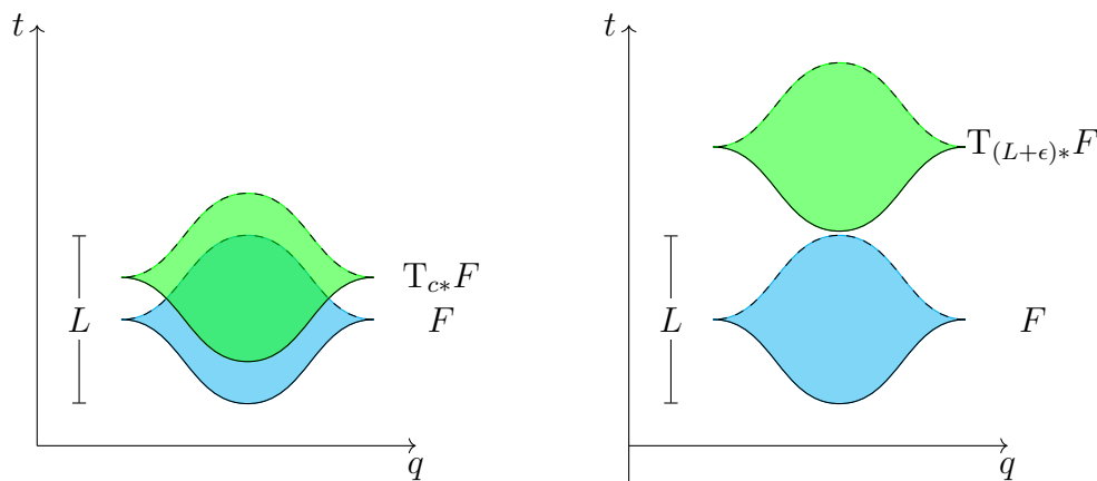
FIGURE 0.1. Considérons le faisceau constant F = \mathbb{K}_Z , où Z est l'ensemble localement fermé bleu. Puisque la frontière de Z est la projection frontale du noeud legendrien trivial, nous avons que SS(F) est la conification du noeud legendrien trivial en J^1\mathbb{R} . De plus, nous définissons L comme étant la longueur de la seule corde de Reeb. On peut montrer que \tau_c(F) = 0 pour c > L et \tau_c(F) \neq 0 pour 0 \leq c < L . De cette façon, nous trouvons la longueur de la corde de Reeb.
